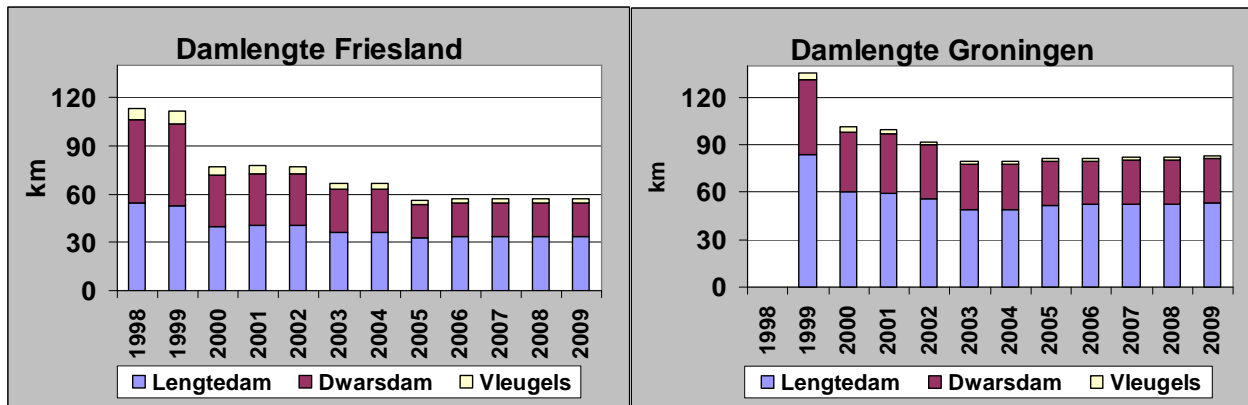
Figuur 3.2. Bestand aan rijshoutdammen in de kwelderwerken (bron: legger RWS).
