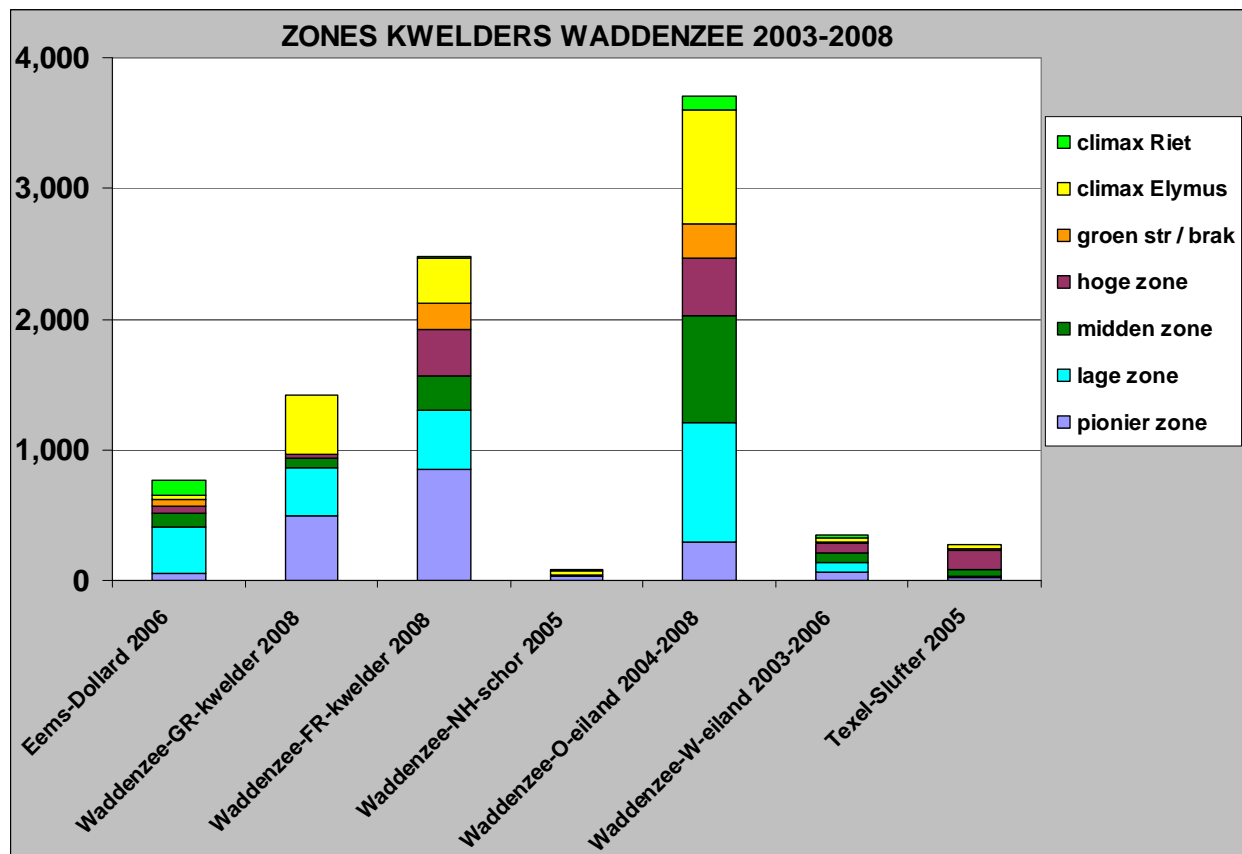
Figuur 1.2. Areaal pionierzone en kwelderzones in ha op basis van vegetatiekaarten RWS-DID 2003-2008 (methode KRW-classificatie in Dijkema et al. 2005). Areaal vastelandskwelders = boerenkwelders + kwelderwerken (zonder zomerpolders). Pionierzones van luchtfoto's; Waddenzee bedekking > ca. 5 %; pionierzones ZW Nederland bedekking > 0,1 %. In oostelijke eilanden zit in 2006 een 700 ha groter gekarteerd polygoon voor de Boschplaat.
