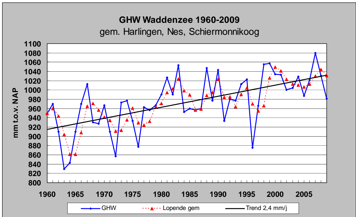
Figuur 2.4. Jaargemiddelde hoogwaters voor de kwelderwerken van 1960-2009.
