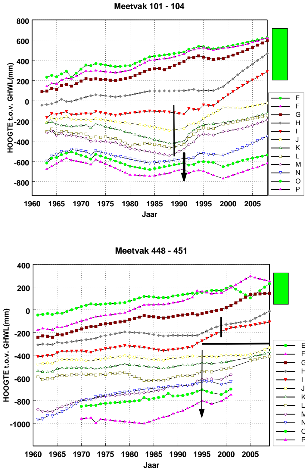
Figuur 3.1. Effect van tussendammen in de pionierzone (1989, 1995, 1999) en van afstoten van buitenste bezinkvelden (1991, 1995) op de hoogteligging in de meetvakken 101 en 448. Legenda zie bijlage 2.
